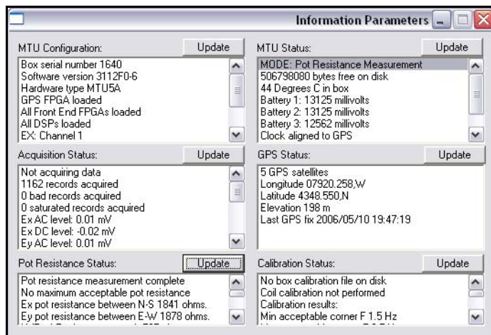
Fig. 3-4: The Information Parameters dialog box.
